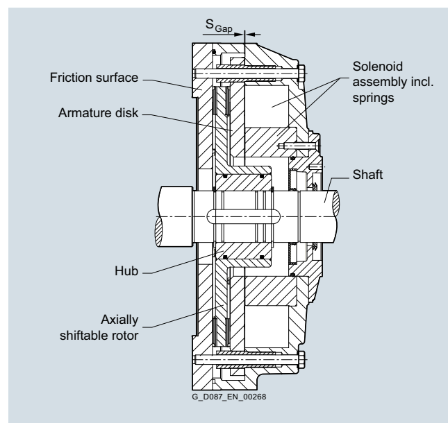
Fig. 11/33 Brake FDX
