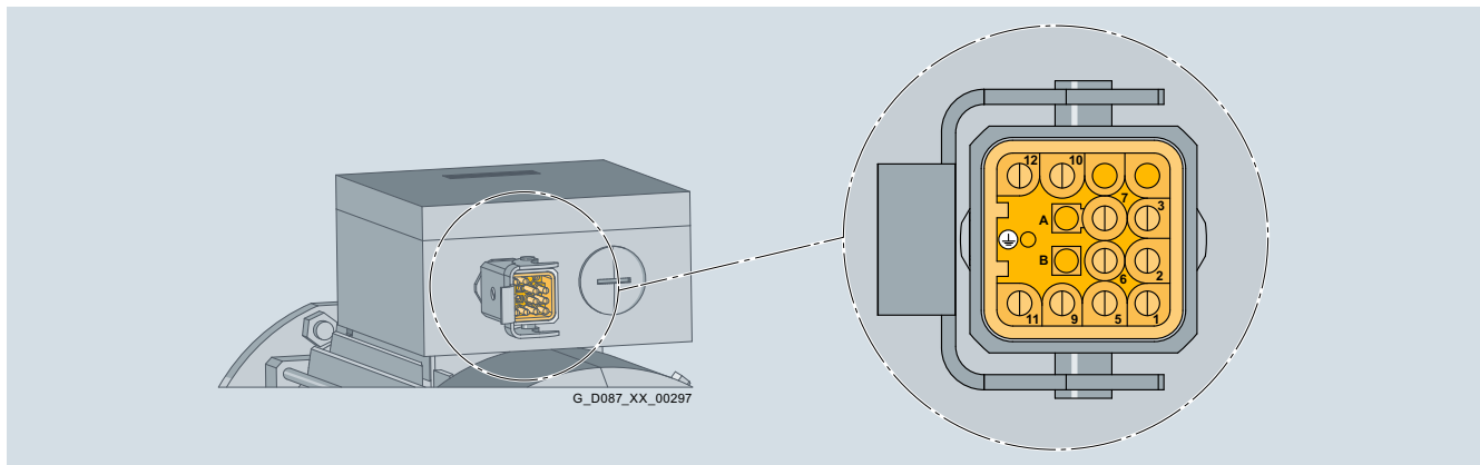
Fig. 11/30 HAN Q12 motor plug with pin assignments
