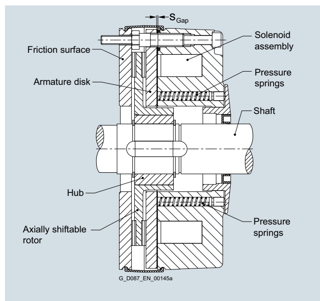
Fig. 11/32 Brake L
